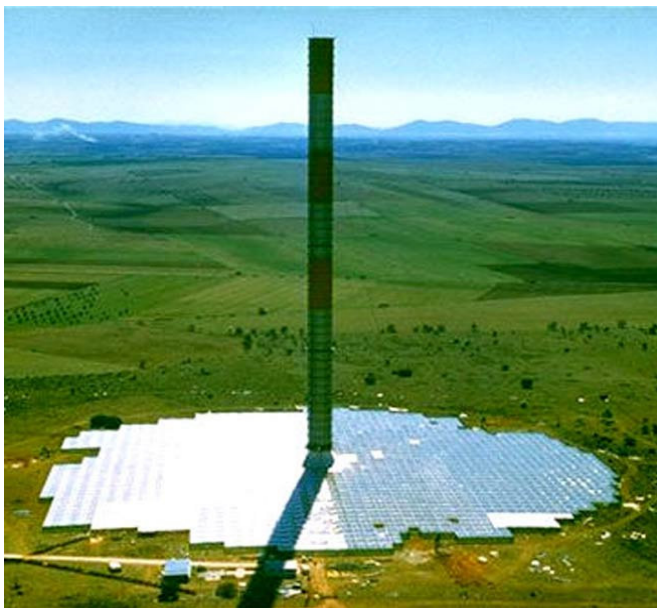
Figura 2 - prototipo di torre solare a ventilazione.
