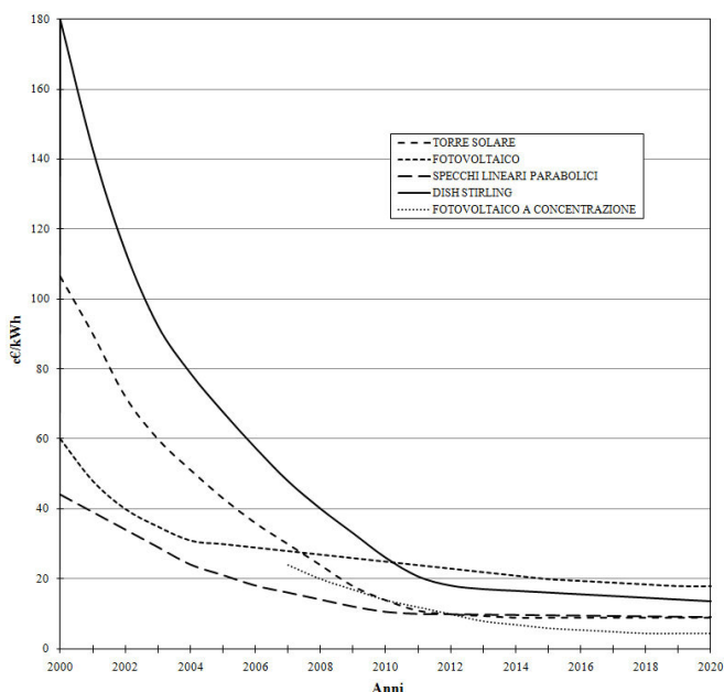
Figura 13 - previsione dell'andamento del LEC dei vari sistemi solari.
