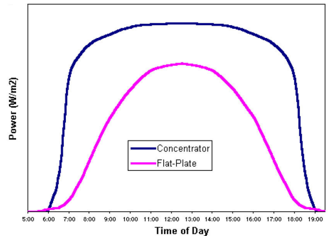
Figura 6 - confronto sulla potenza raccolta tra sistema fotovoltaico tradizionale ( Flat - Plate ) ed a concentrazione.
