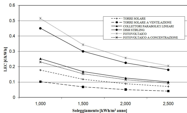
Figura 12 - andamento del LEC al variare del soleggiamento \beta .
