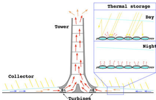
Figura 3 - funzionamento di torre solare a ventilazione.
