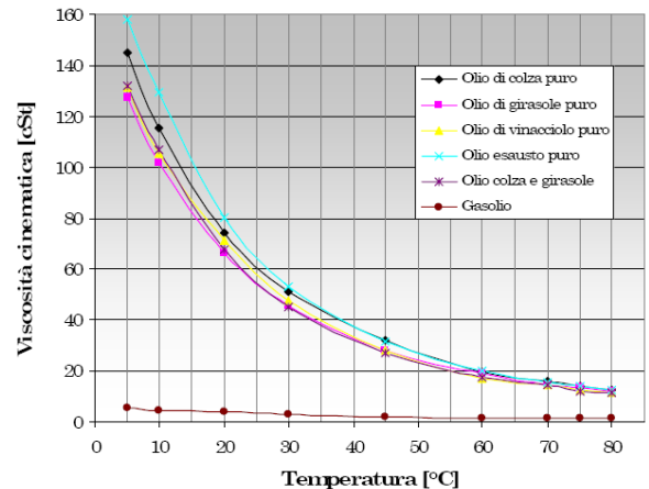
Figura 2: Confronto tra la viscosità cinematica degli oli e quella del gasolio.
